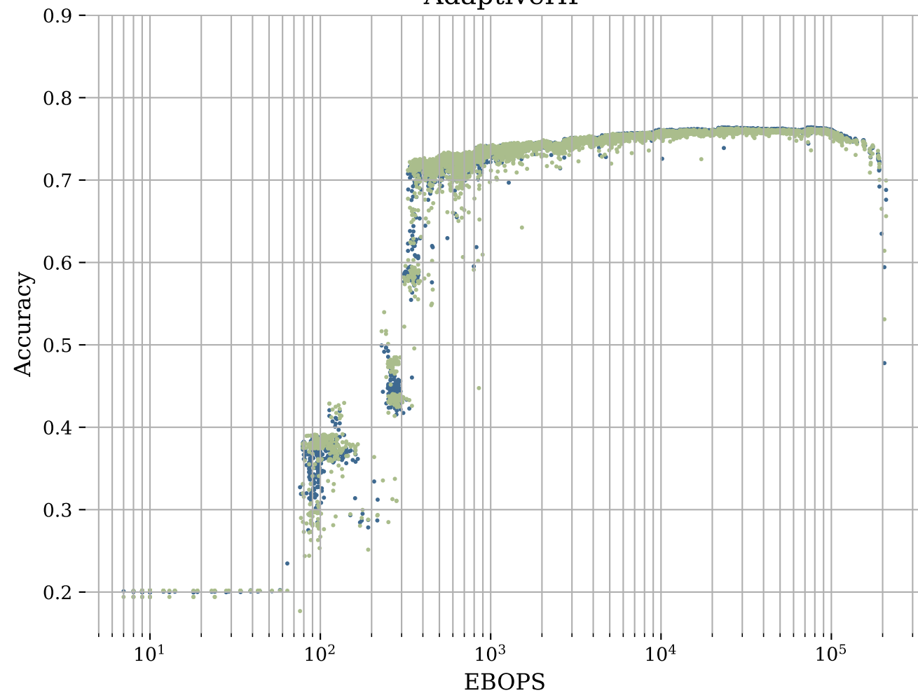
AdaptiveHP
