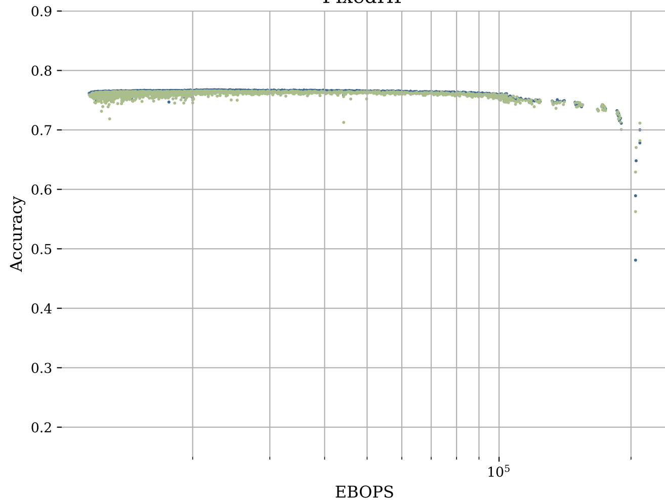
FixedHP
